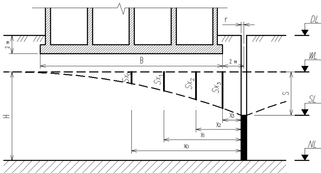
Рис.1. Расчетная схема к задаче 6
